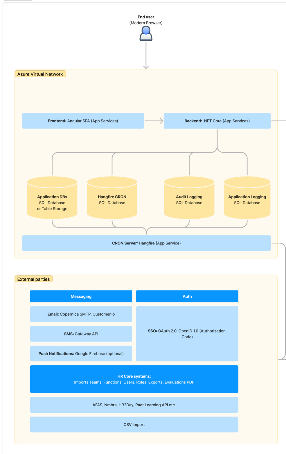
Afbeelding 1: Architectuur
